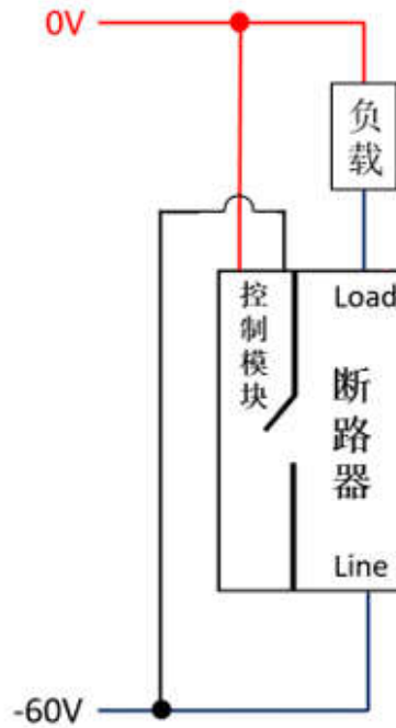
接线图
